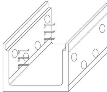
圖 4.4-2 電纜溝電纜分匯部構造示意圖
