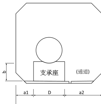
圖 3.5-2 瓦斯幹管管道斷面示意圖
