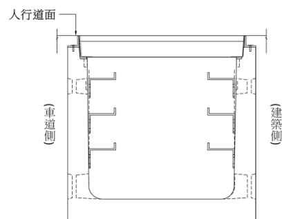
圖 3.4-4 電纜溝示意圖
