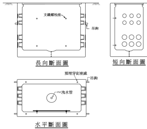
圖 3.4-5 纜線管路手孔示意圖
