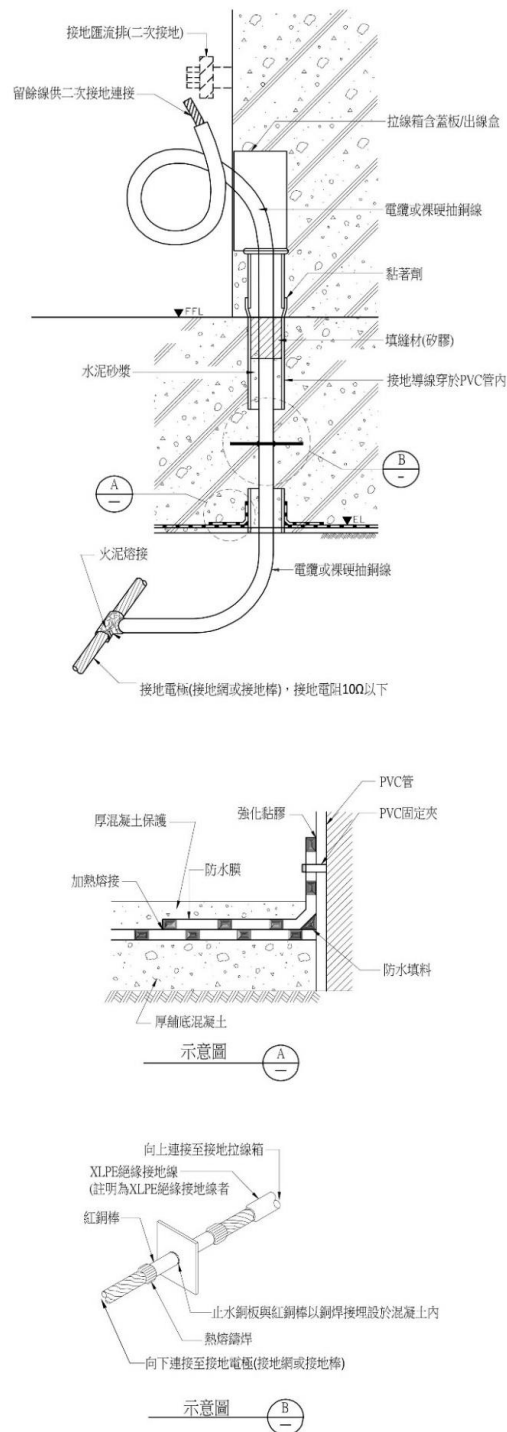
圖 4.1-4 接地系統止水示意圖
