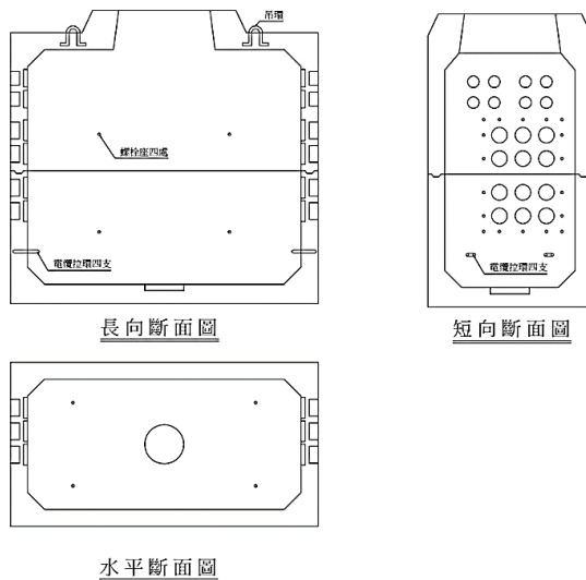
圖 3.4-5 纜線管路手孔示意圖
