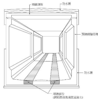
圖 4.3-2 版式預鑄構件示意圖
