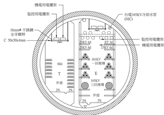
圖 3.4-2 圓形共同管道斷面配置示意圖
