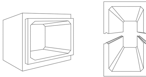
圖 4.3-1 箱式預鑄構件示意圖
