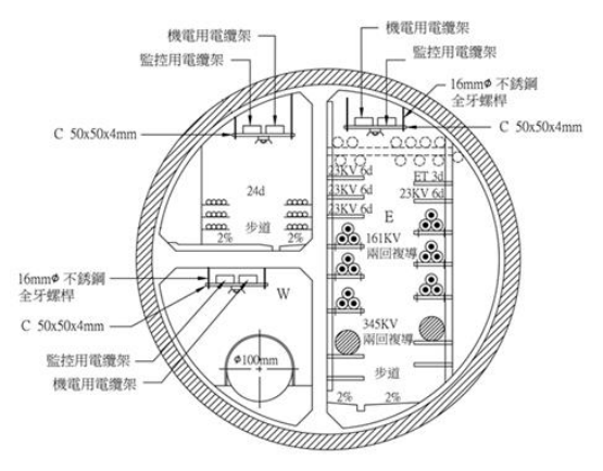
圖 3.4-1 箱型共同管道斷面配置示意圖
