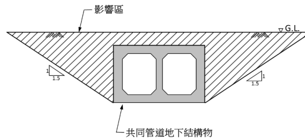
圖 4.1-1 地下結構物之影響區示意圖
